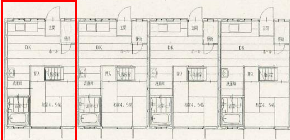
<1階平面図> ※8戸タイプ
