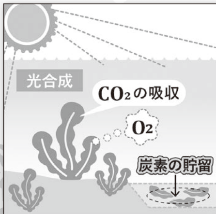
図 海藻・海藻によるCO 2 吸収と炭素貯留のイメージ
