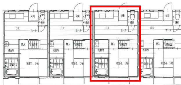
<1階平面図>
