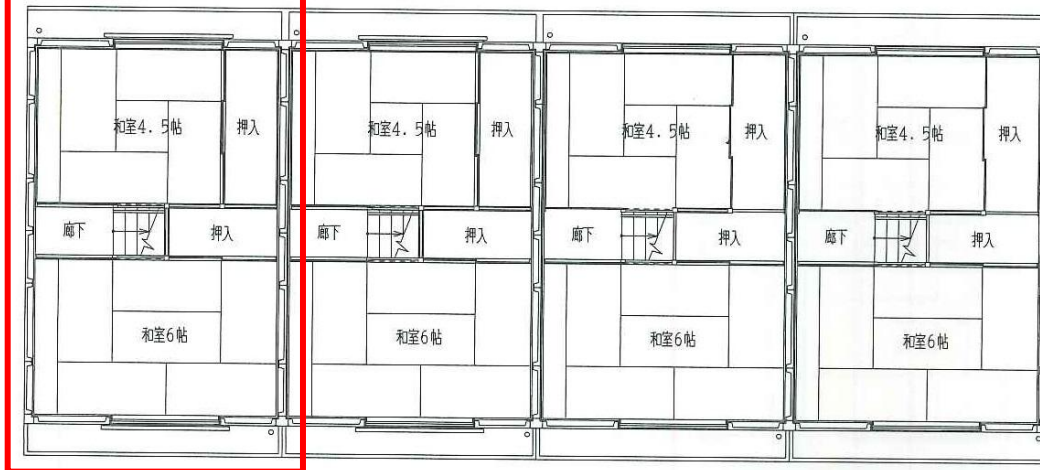
<2階平面図>
