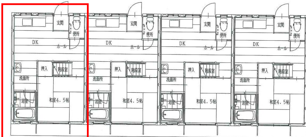
<1階平面図>
