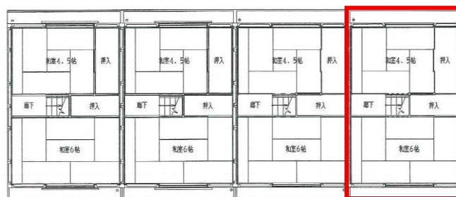
<2階平面図>
